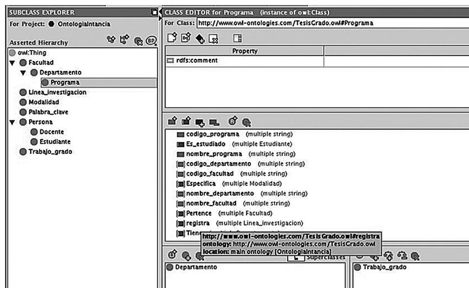
Figura 10. Clase Programa
