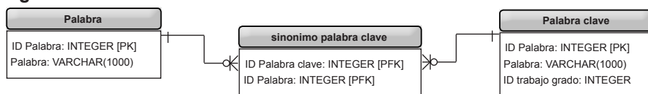
Figura 6. Palabra clave.
