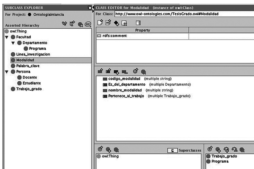
Figura 12. Superclase modalidad
