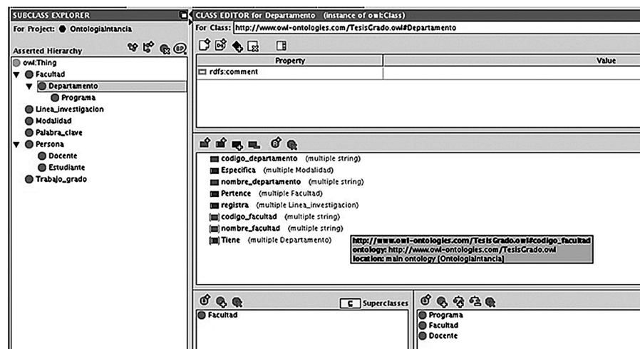
Figura 9. Clase Departamento
