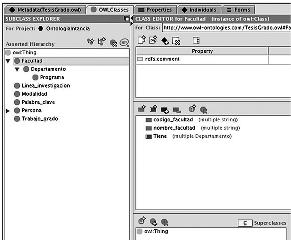
Figura 8. Superclase Facultad
