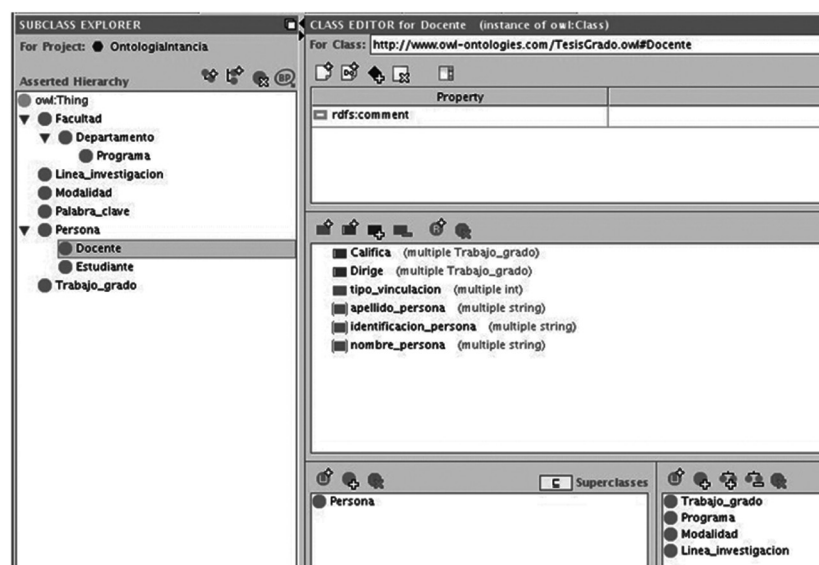
Figura 15. Clase docente
