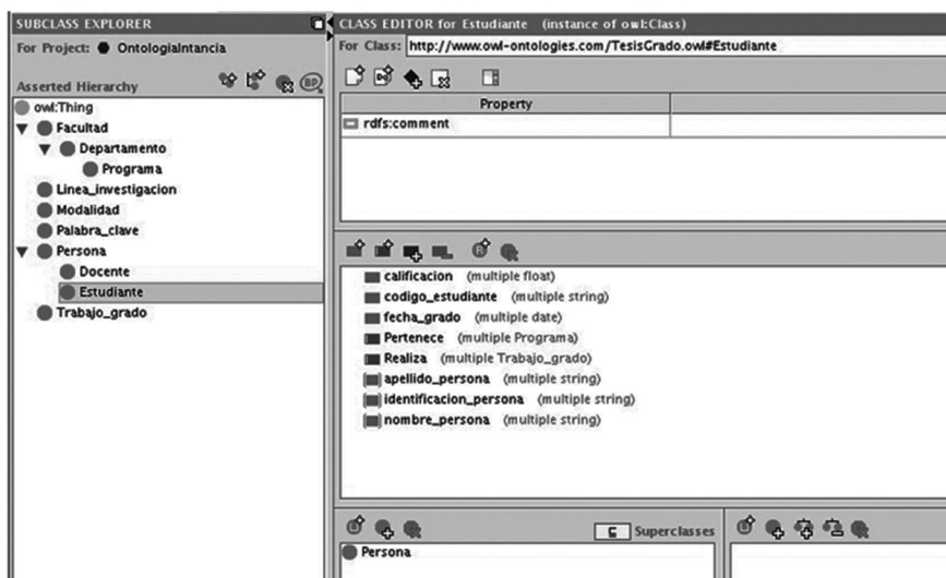
Figura 16. Clase estudiante
