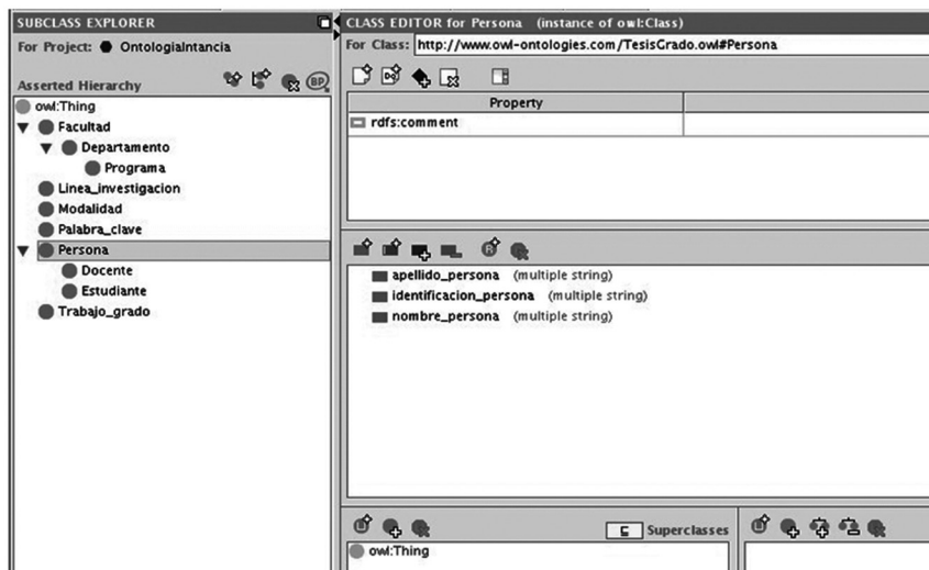
Figura 14. Superclase persona.
