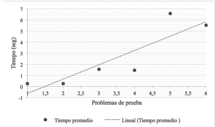
Figura 5. Tiempo promedio de las soluciones obtenidas para cada problema de prueba
