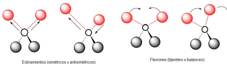
Figura 10. Algunas vibraciones típicas de los átomos
