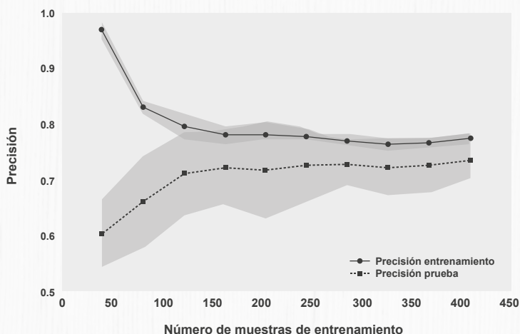
Figura 3. Curva de aprendizaje, modelo de regresión logística
