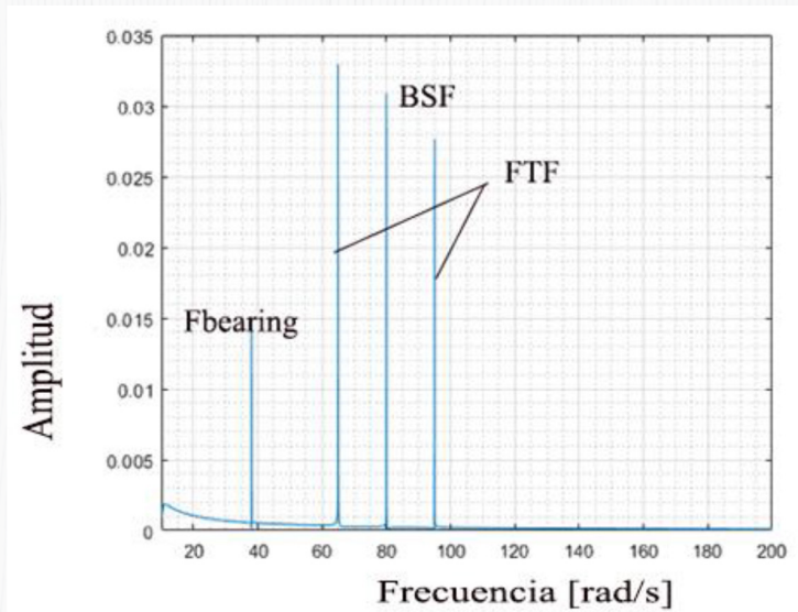
Figura 10. Espectro en frecuencia del deterioro en los elementos rodantes del rodamiento
