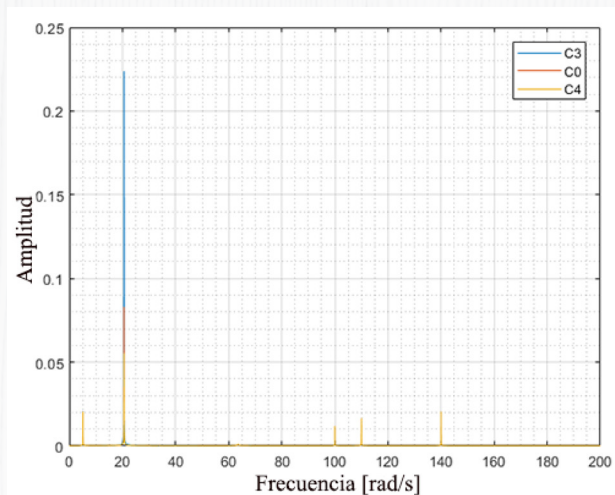
Figura 11. Espectro en frecuencia de la falla en el engranaje variando los parámetros
