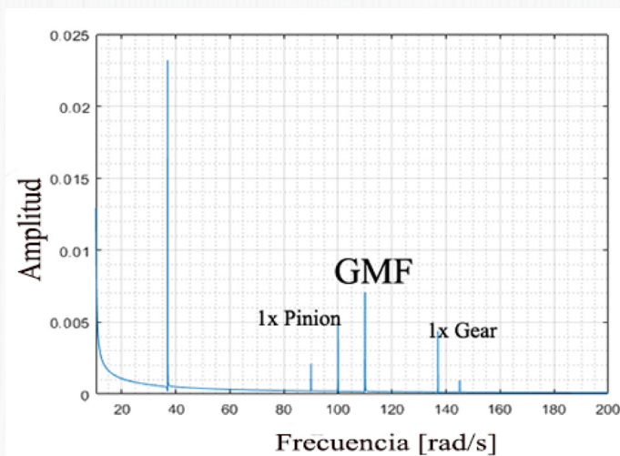
Figura 7. Espectro en frecuencia con la falla desgaste en el diente del engrane
