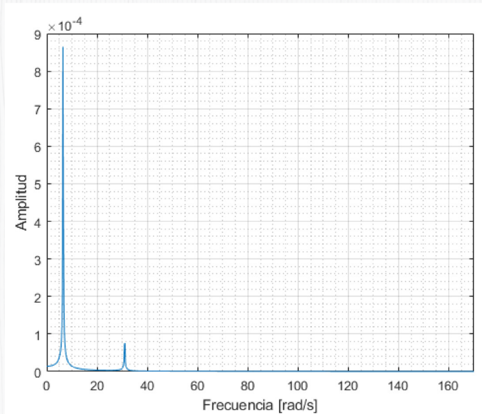
Figura 6. Espectro en frecuencia del comportamiento del sistema
