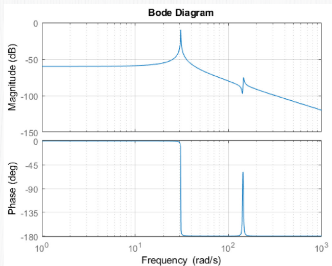
Figura 4. Diagrama de Bode del sistema de 3 GDL
