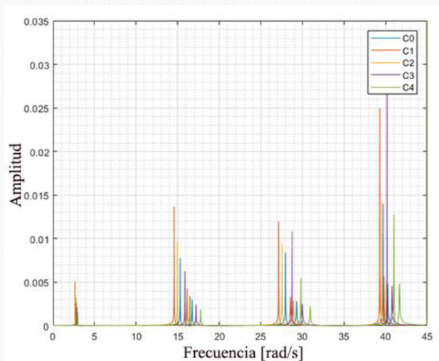
Figura 12. Espectro en frecuencia de la falla en el rodamiento variando los parámetros
