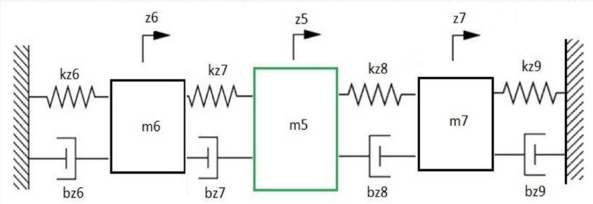
Figura 1. Representación grados de libertad axiales
