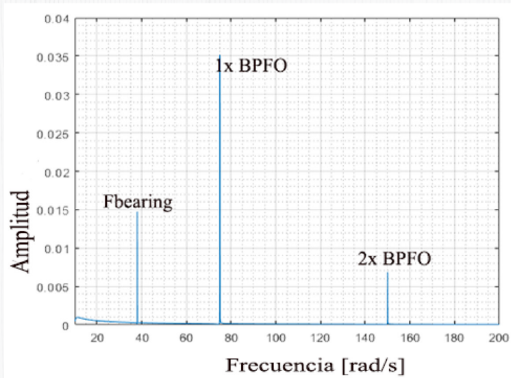
Figura 9. Espectro en frecuencia del deterioro en la pista exterior del rodamiento
