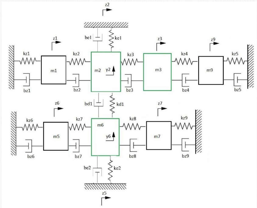
Figura 2. Representación del acoplamiento de los ejes
