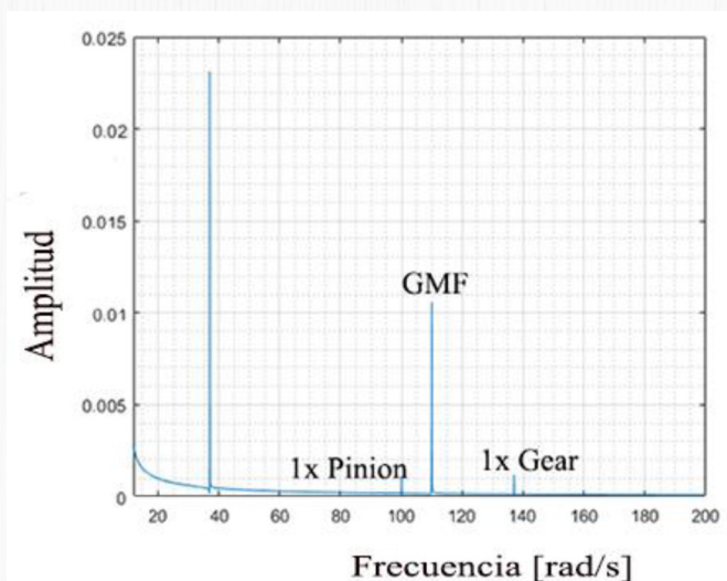
Figura 8. Espectro en frecuencia con la falla sobrecarga de los dientes de engrane
