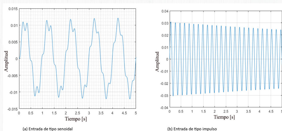
Figura 5. Respuesta temporal del sistema ante distintas entradas
