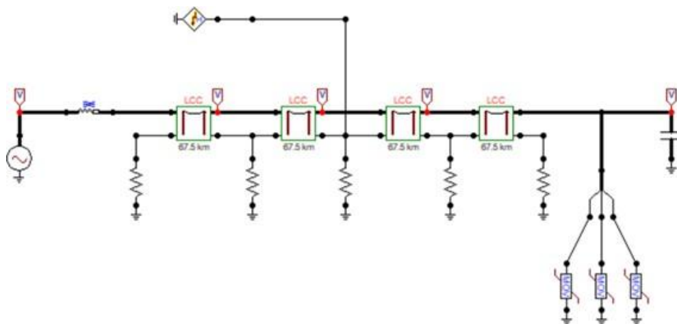
Figura 3. Modelo en ATPDraw
