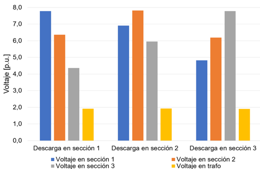
Figura 5. Voltajes en la línea en diferentes lugares de descarga con DPS
