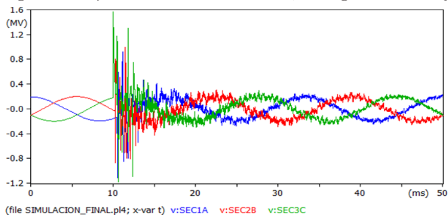
Figura 4. Voltaje en las tres secciones con DPS, descarga en la sección (a) 1 (b) 2 (c) 3
