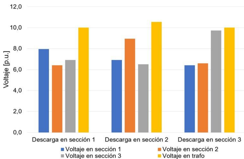
Figura 6. Voltajes en la línea en diferentes lugares de descarga sin DPS
