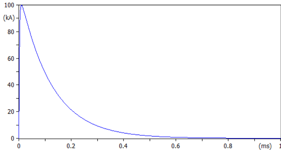
Figura 1. Forma de onda de la corriente del rayo usada
