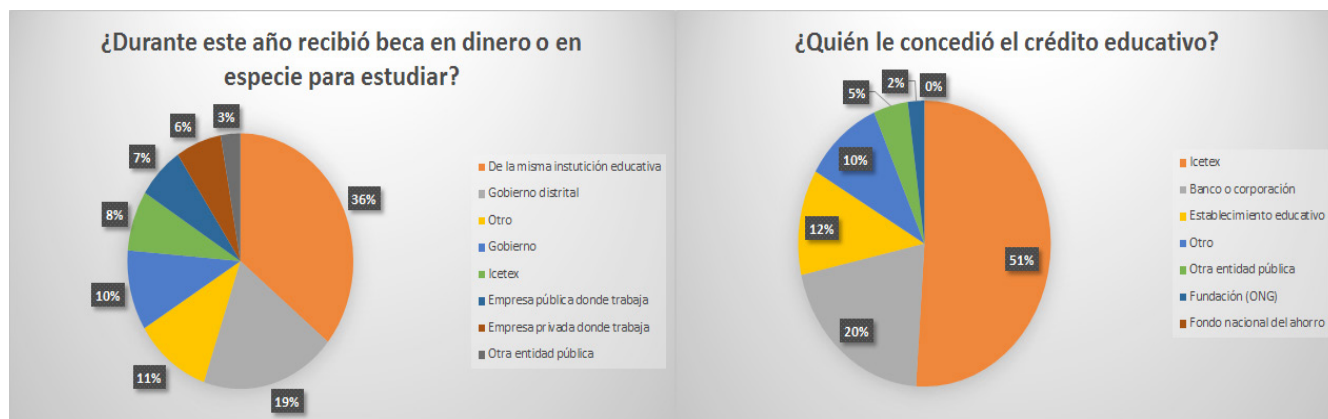
Figura 2. Preguntas P8610 y P6202
